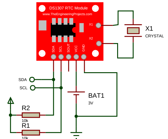
U1 DS1307
