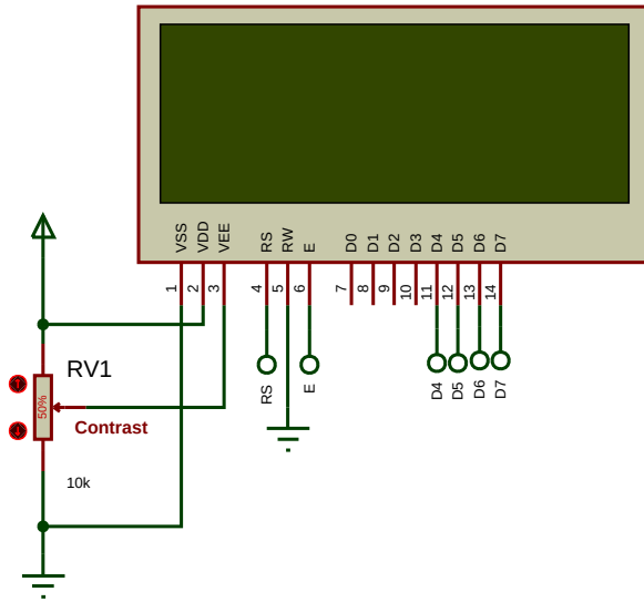
LCD1 LM044L
